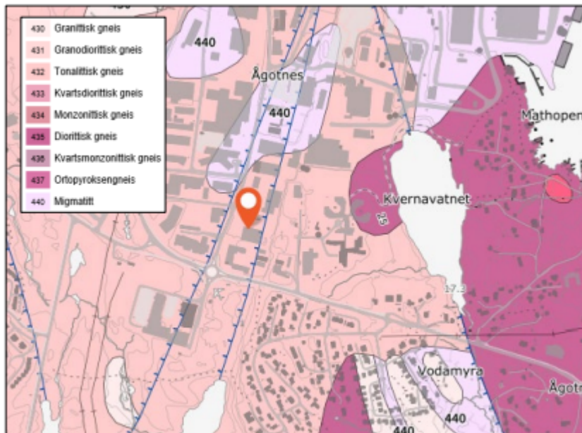
Figur 5 Berggrunnskart fra NGUs Nasjonale berggrunnsdatabase ( https://geo.ngu.no/kart/berggrunn_mobil/ ).
