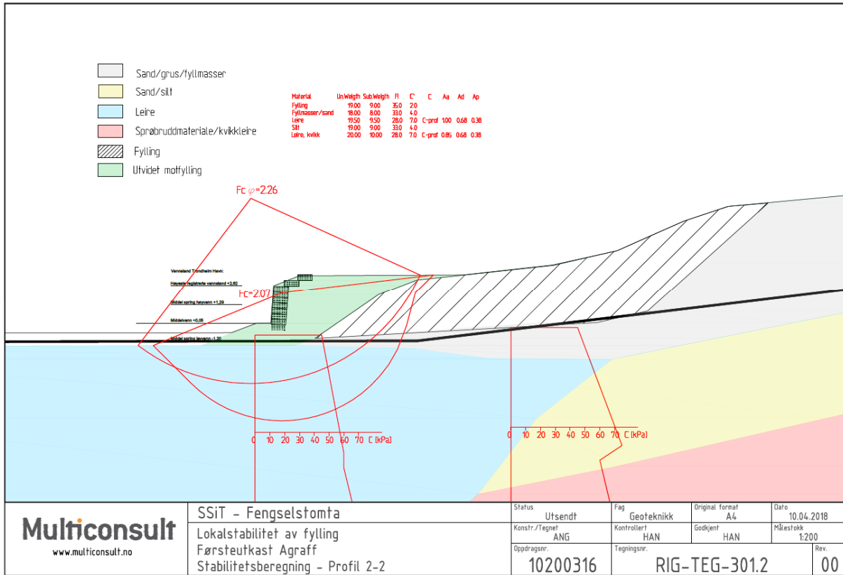
Figur 6 Prinsippkisse av profil 2.
