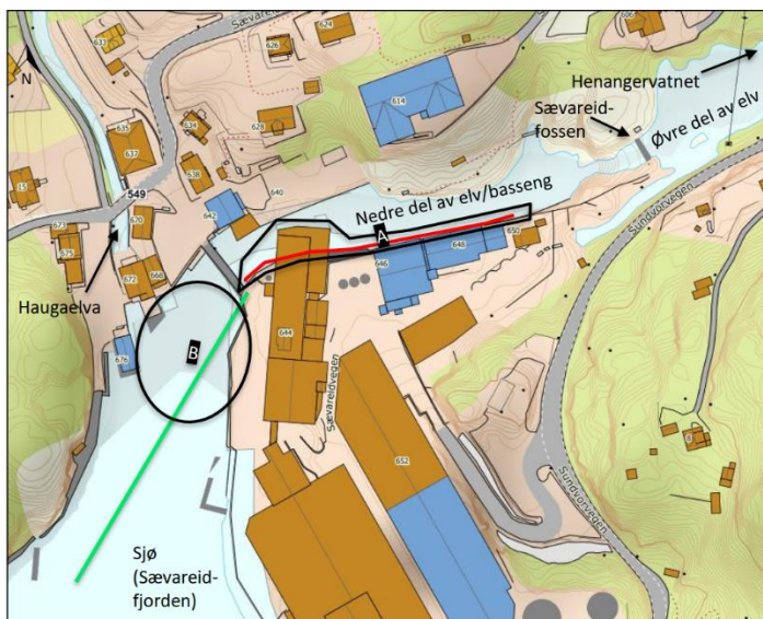
Figur 1 Oversiktskart som viser lokaliseringsområdet for tiltaksområde A i basseng/nedre del av elven (svart figur) og tiltaksområde B sør for broen (svart ellipse). Rød linje viser ny betongmur, mens grønn linje viser trase sjøledninger
