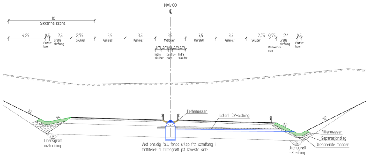
Figur 4 Prinsipp infiltrasjonsgrøfter.
