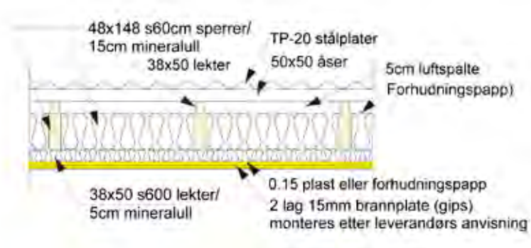
FIGUR 18 Detalj fra takkonstruksjon
