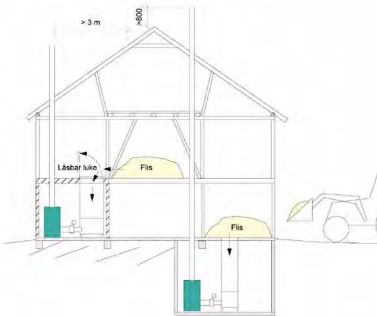
FIGUR 6 Enkelt anlegg – manuell fylling
