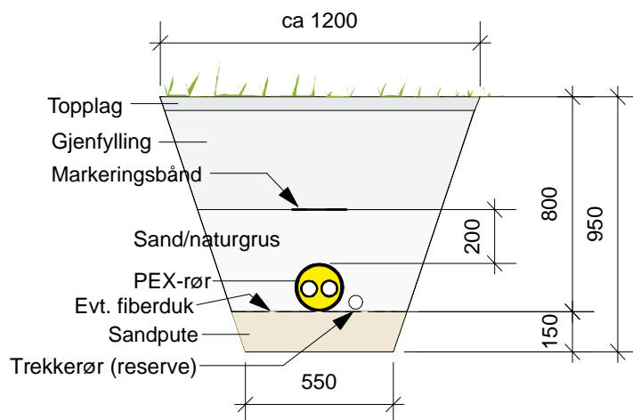
FIGUR 24 Skisse av grøft
