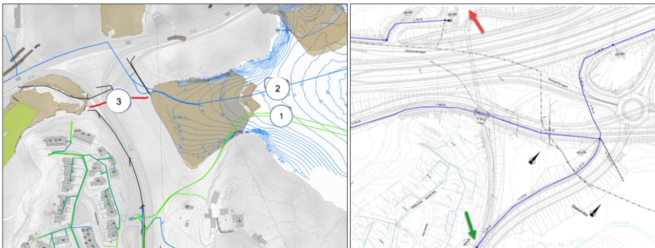
Figur 22 - Omlegging av vannledning ved Stekervika, bilde til venstre er eksisterende situasjon der 1 er Spillvannsledning OID 5737/ 5393, 2 er Vannledning OID 5519/ 5488 og 3 er kulvert for bekk. Bildet til høyre er ny situasjon for vannledning.
