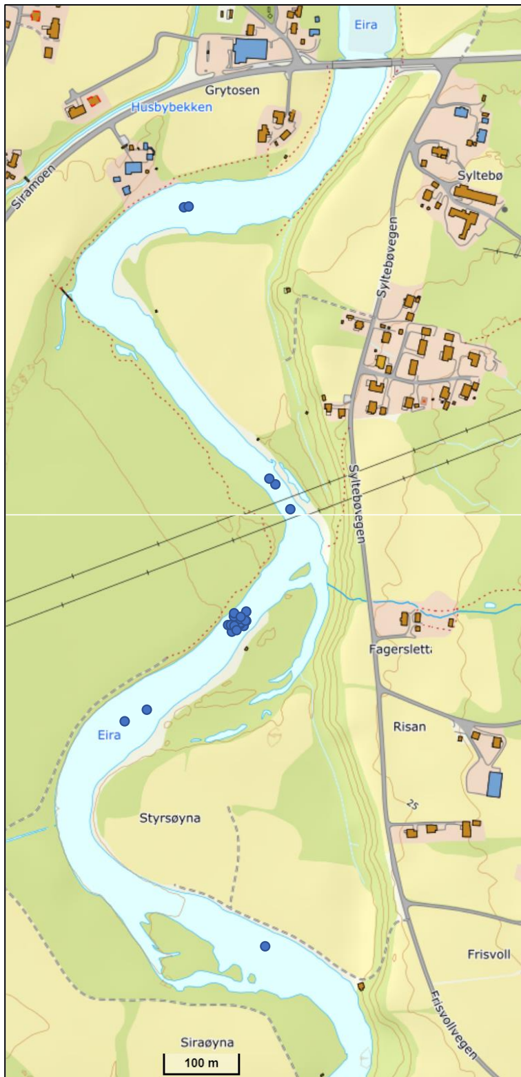
Figur 13. Posisjonen til levende elvemusling som ble observert under fritellingene i Eira i oktober 2021 (jf. figur 12 og vedlegg 7.2). Da det er relativt korte strekninger som er undersøkt (små arealer) på hver stasjon, er det forventet å finne spredte muslinger også i andre deler av elva på denne strekningen.
