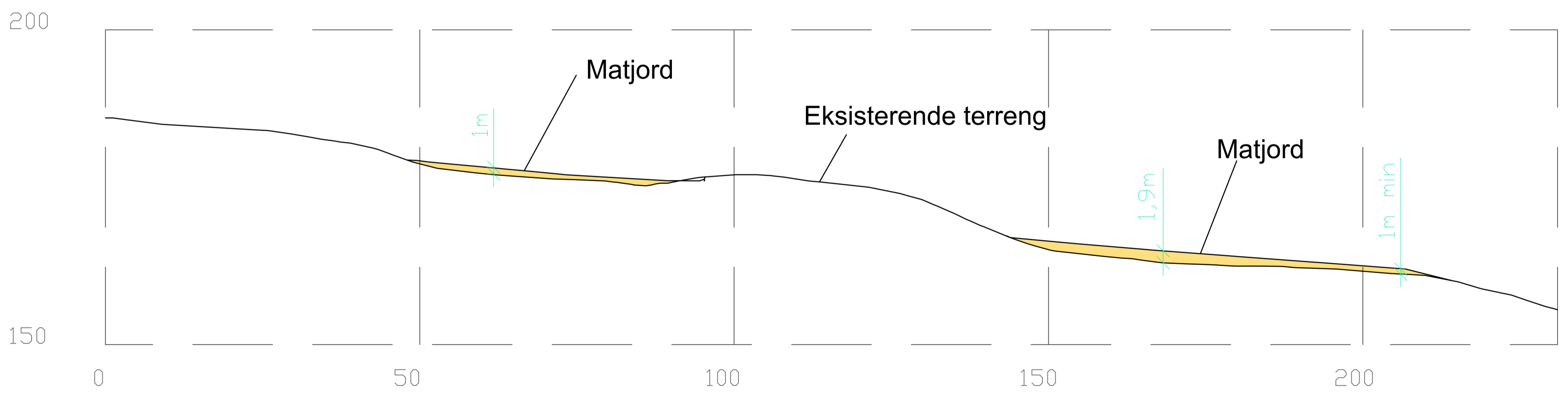
Snitt B-B` M 1:500
