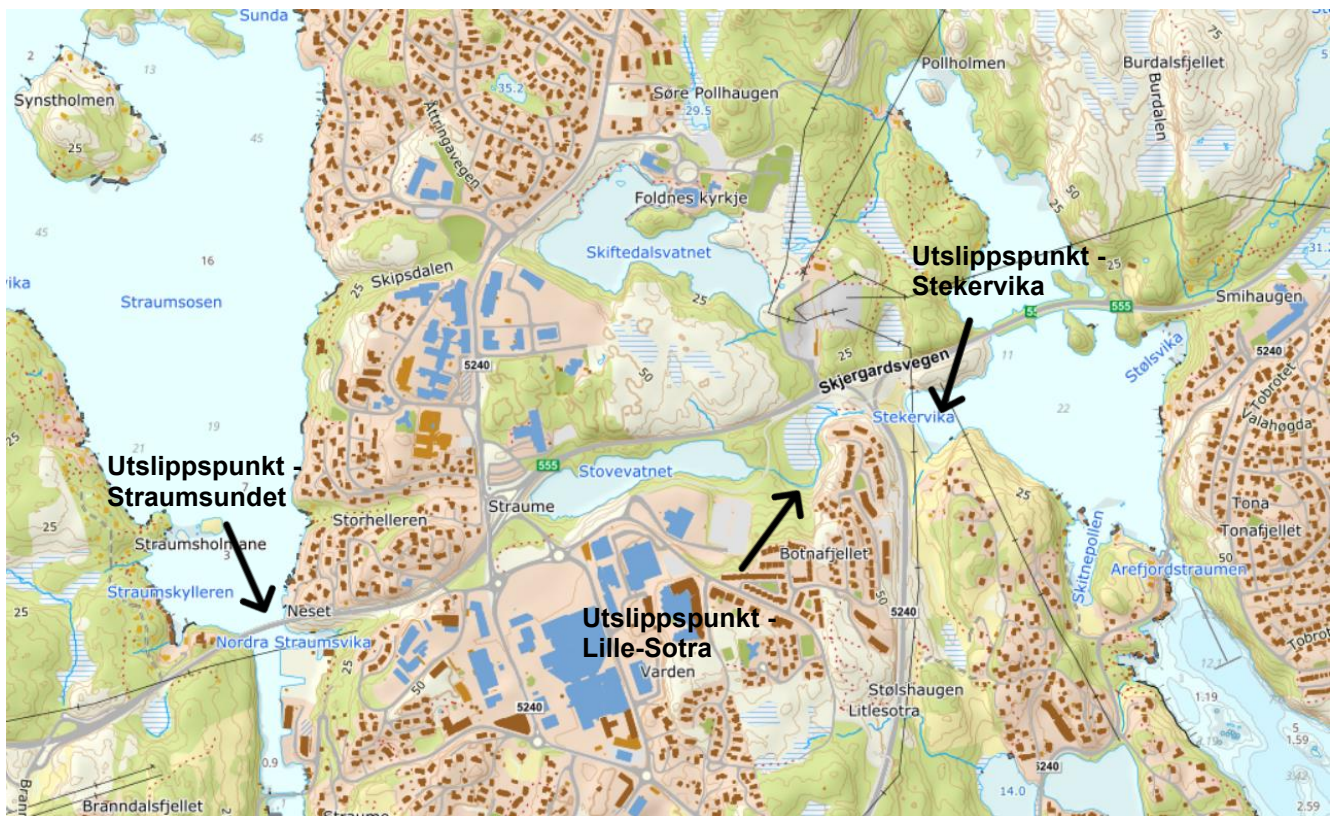
Figur 2: Figuren viser omtrentlige utslippspunkter for tunnelvann fra Straumetunnelen. I anleggsfase skal tunnelvann renses og slippes ut i elva Lille-Sotra eller i sjø ved Stekervika. I driftsfasen skal tunnelvann renses og slippes ut i Straumssund.
