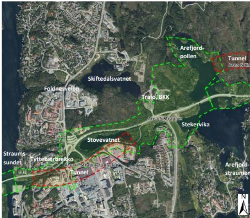
Figur 3: Oversiktskart hentet fra prosjektets GIS-modell som viser strekning A4 Straumetunnelen. Grønn stiptet linje markerer dagsoner og rød stiptet linje markerer tunnel. Kilde: Kartverket, Geodata.
