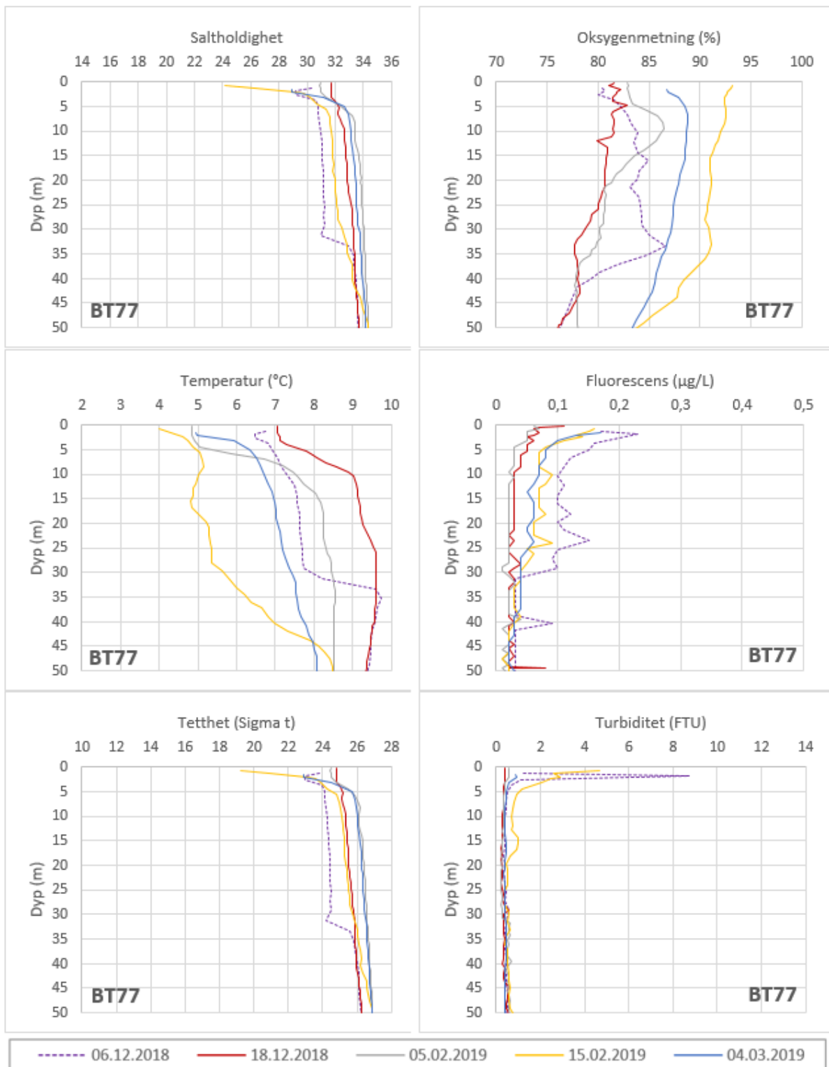
Figur 9: Saltholdighet (øverst t.v.), temperatur (midt t.v.), tetthet (nederst t.v.), oksygenmetning (øverst t.h.), fluorescens (midt t.h.), og turbiditet (nederst t.h) i de øverste 50 m på stasjon BT77 (stasjonen er 88 m dyp).
