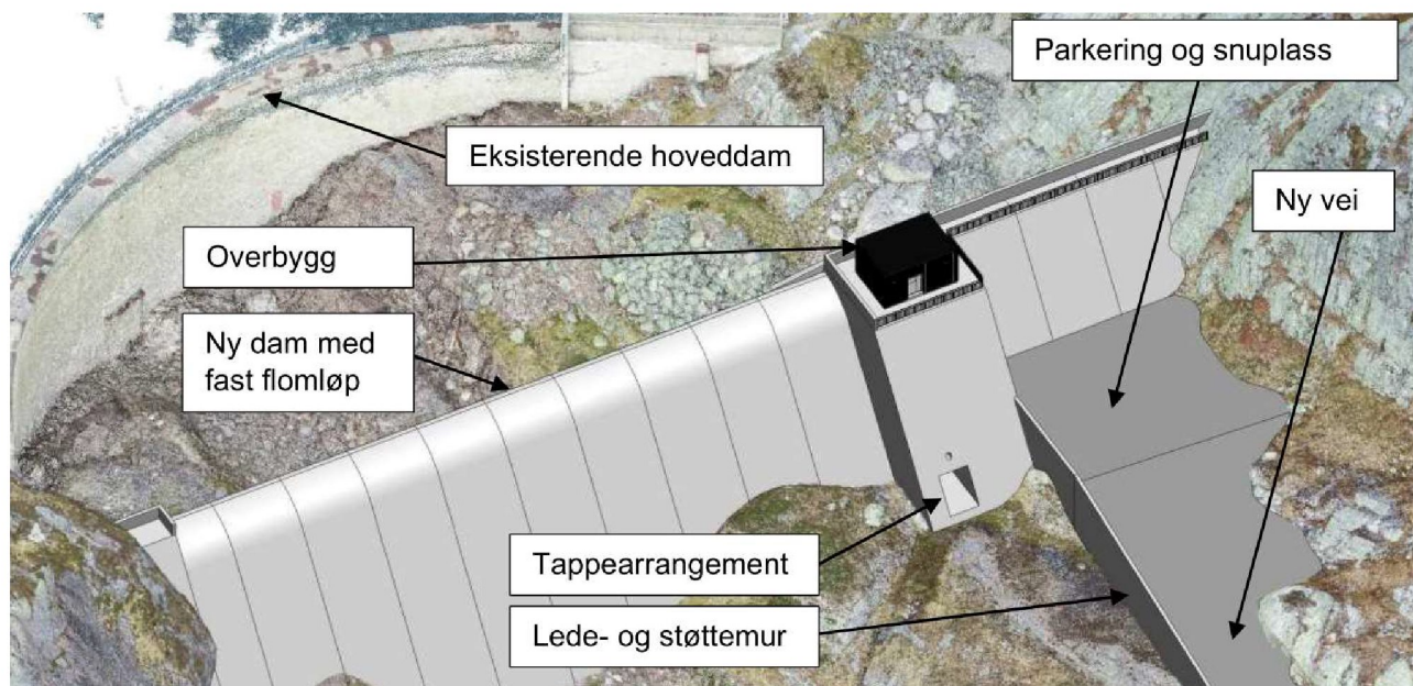
Figur 2-2: Planlagt ny dam nedstrøms eksisterende hoved- og sperredam. Snuplass og parkering med kombinert lede- og støttemur til høyre.
