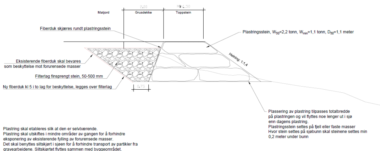
Figur 1: Tegning av profil og beskrivelse av metoden for utfylling i sjø i forbindelse med utbedring av erosjonssikring/plastring ved Jadarholm. Kilde: søknadsvedlegg
