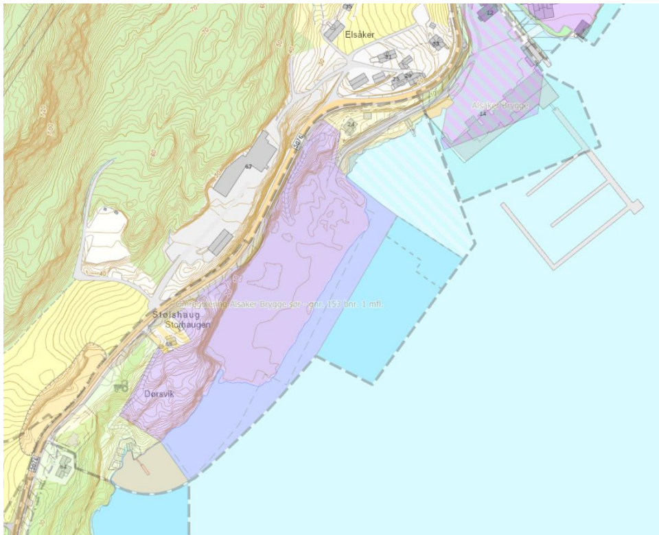
Figur 1 Utfyllingen er vist med lilla farge - Kilde Kystinfo med reguleringsplan inntegnet
