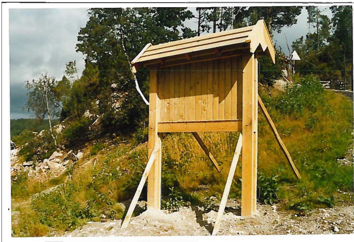
Figur 22. Oppslagstavle laga etter DN-standard, Øvstbøen.
