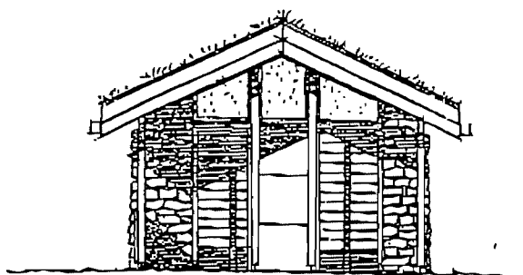
FASADE SYD
