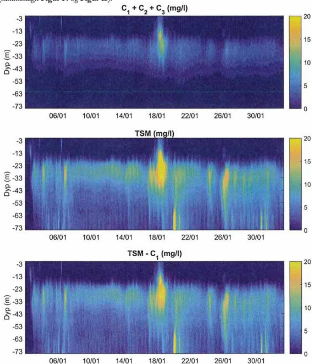
Figur 14. Partikkelkonsentrasjon på stasjon 2. Øverst vises summen av de tre minste partikkelklassene med kornstørrelse mindre enn 16 \mu\text{m} . I midten vises summen av alle de ni partikkelklassene. Nederst vises effekten av å fjerne partikler mindre enn 4 \mu\text{m} . Kornfordeling med mye finstoff er brukt (jamfør Figur 9 ).
