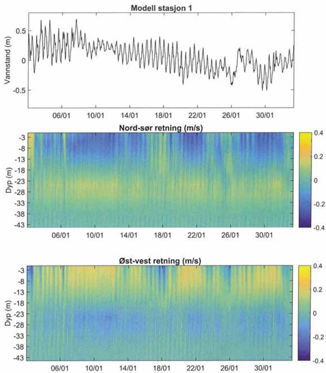
Figur 8. Beregnet vannstand og strøm på modell stasjon 1. Tidsperioden som er modellert er januar 2014.
