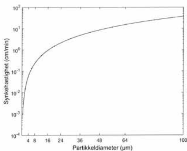
Figur 10. Synkehastighet etter Stokes lov.
