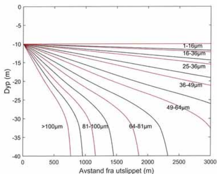
Figur 11. Beregnede partikkelbaner for partikler med forskjellig kornstørrelse, basert på målt strøm (svarte linjer). De røde linjene viser de samme partikkelbanene når strømhastigheten er redusert til 80 %.
