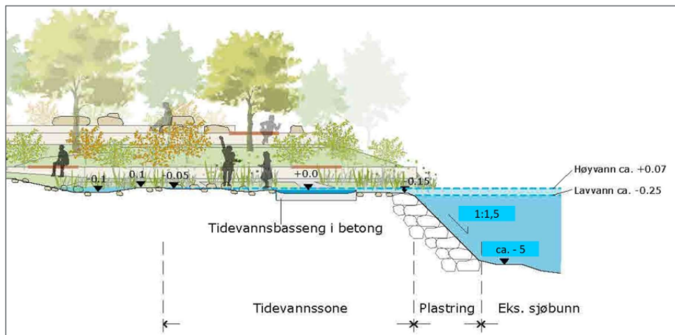
Figur 2: Prinsippkisse for møte mellom land og sjø ved Sjøkanten park. Kilde: Søknadsdokumentasjon.
