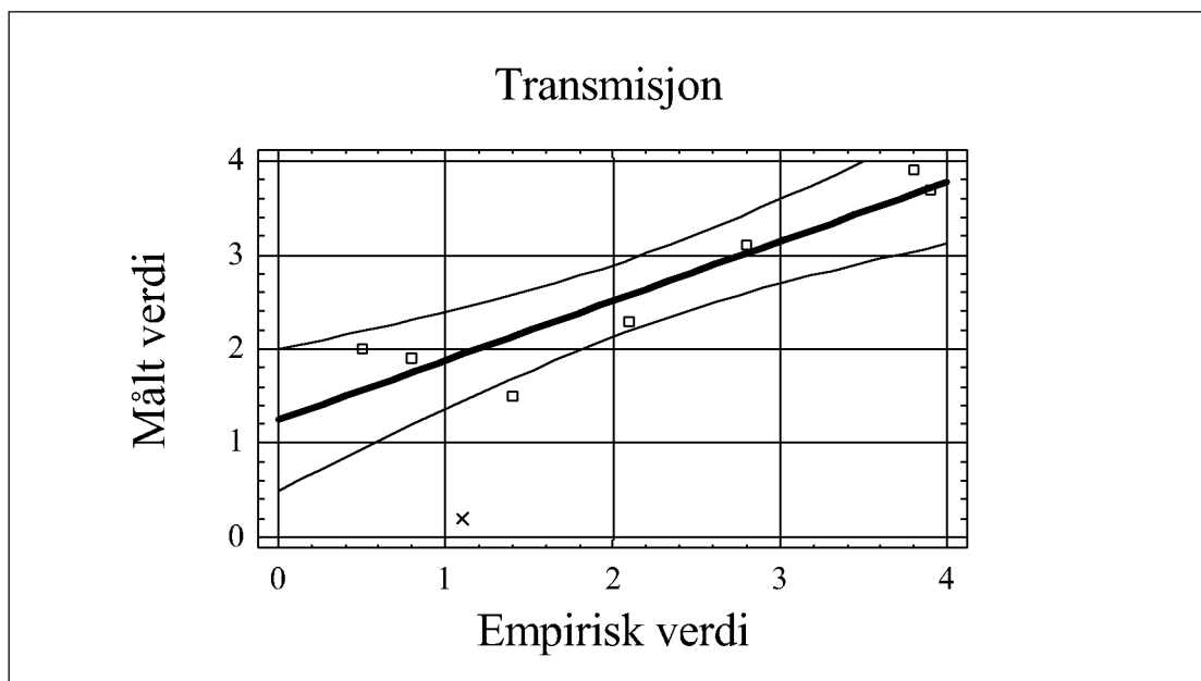
Figur 4.19. Sammenheng mellom empirisk verdi for transmisjon og verdier som ble målt i Hannevikbukta. Korrelasjonskoeffisienten for den lineære regresjonslinja er r^2=0.852 . Tynnere linjer omkring regresjonslinja viser 95% konfidensintervall. Måling angitt med "x" er ekskludert fra beregningene.
