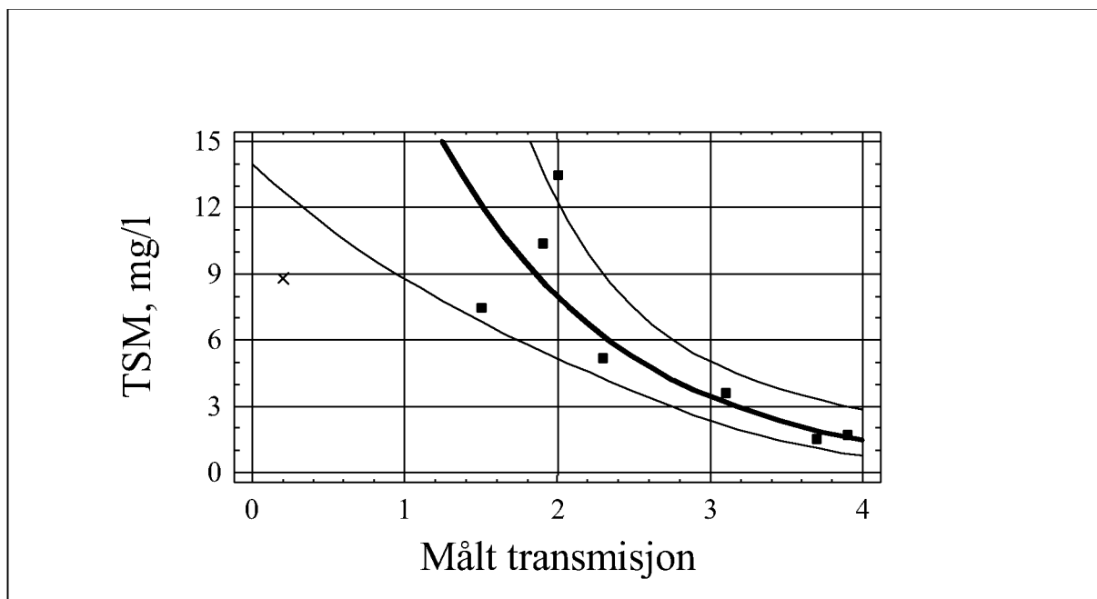
Figur 4.20. Sammenhengen mellom målt transmisjon og konsentrasjon av TSM i Hannevikbukta. Korrelasjonskoeffisienten for den eksponensielle regresjonslinja er 0.857. Tynnere linjer omkring regresjonslinja viser 95% konfidensintervall. Måling angitt med "x" er ekskludert fra beregningene.
