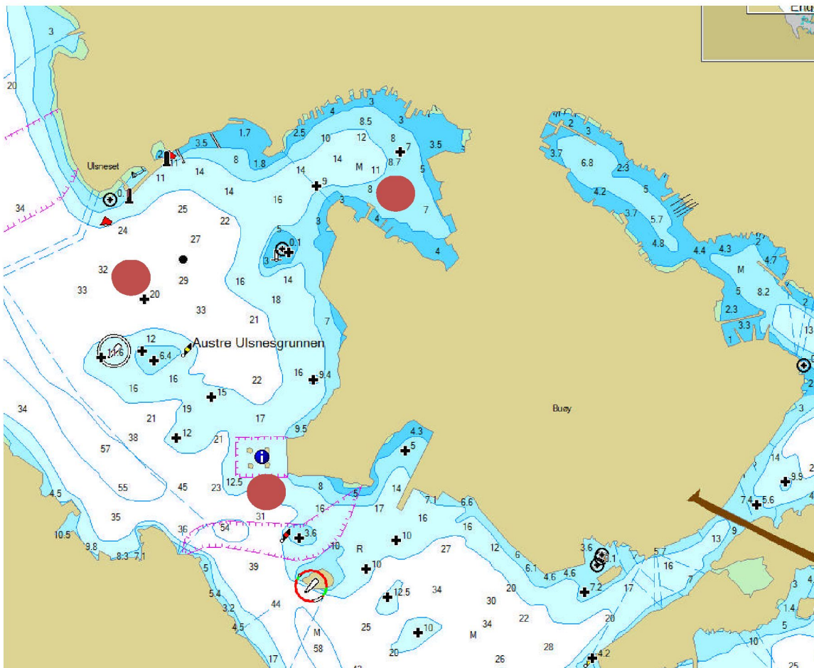
Figur 1: Forslag til plassering av turbiditetsmålere for kontinuerlig turbiditetsmåling
