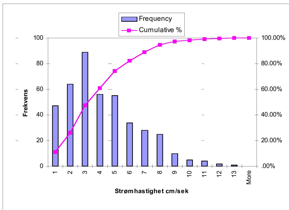
Figur 4.3. Dumpfeltets søndre del. Statistisk fordeling av strømretning og strømhastighet i 17m dyp.
