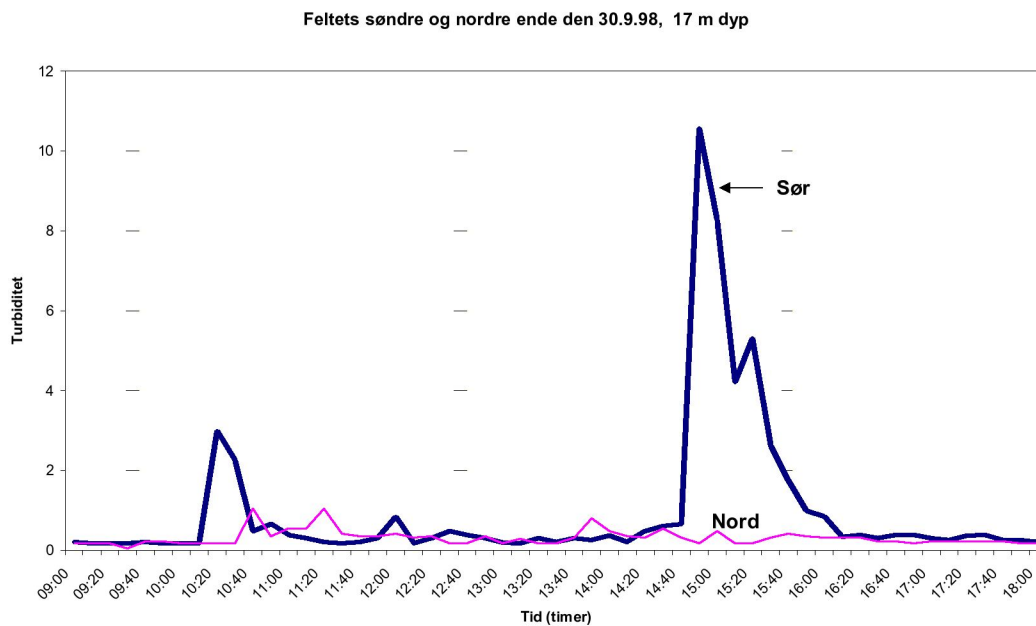
Figur 4.7. Transmisjon målt av strømmålerne på 17 m dyp ved dumpfeltets søndre og nordre ende den 30.9 1998. En partikkelsky etter dumping kl. 10:10 og kl. 14:10 sees tydelig i søndre del.
