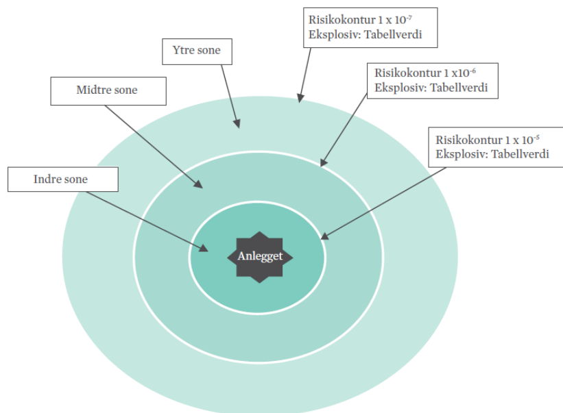
Figur 78: Omsynssoner rundt eit anlegg med innteikning av sikkerheitsavstander/risikokonturer som avgrensar sonene (DSB, 2016).
