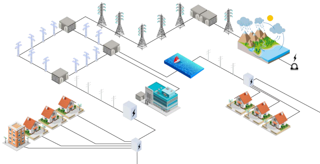
Figur 22: Oppbygning av straumnettet med straumlinjer og transformatorstasjonar i transmisjonsnettet, straumlinjer og transformatorstasjonar i overordna distribusjonsnett (tidlegare regionalnett) og straumlinjer/straumkablar, nettstasjonar og kabelselskap i distribusjonsnettet fram til sluttbrukar (Kjelde: Lyse Elnett).
