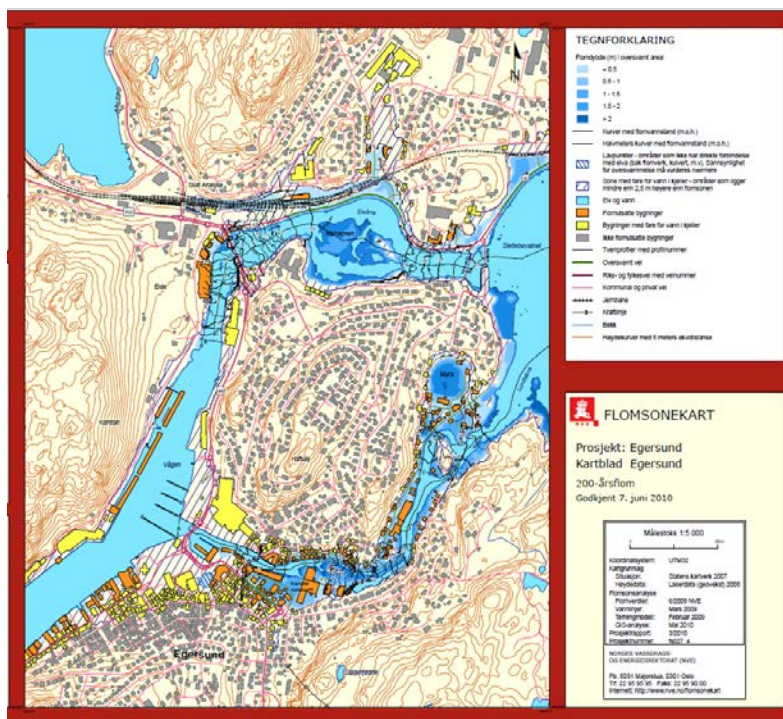
Figur 46: Flaumsonekart, 200-årsflaum i Egersund (NVE, 2010)
