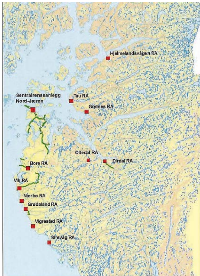
Figur 19: Lokalisering avlaupsanlegga og transportsystemet til IVAR. Reinsanlegg er markert med raudt kvadrat og transportsystem med grøn linje.
