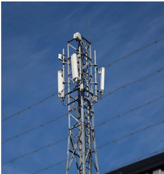
Figur 32: Mast (Foto: Ove Sveinung Tennfjord/Randaberg kommune)
