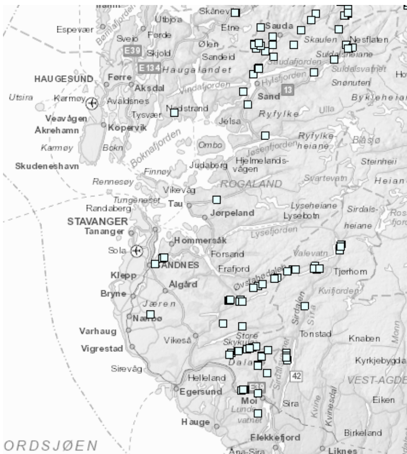
Figur 54: Registrerte snøskred i Rogaland i perioden 05.12.2010 -04.12.2017 (skredregistrering.no)
