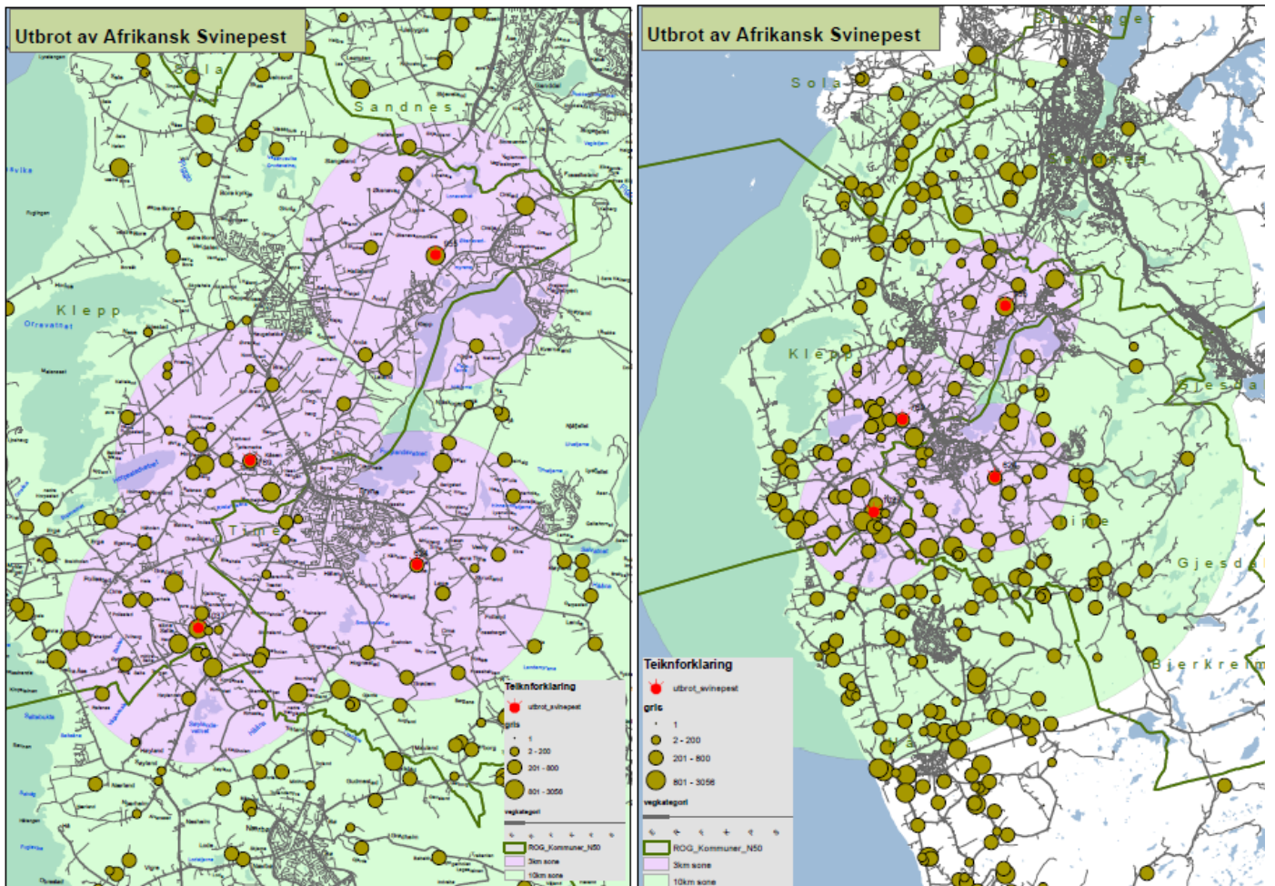
Figur 83: Kart over risiko- og observasjonssone ved utbrot av Afrikansk svinepest på Jæren
