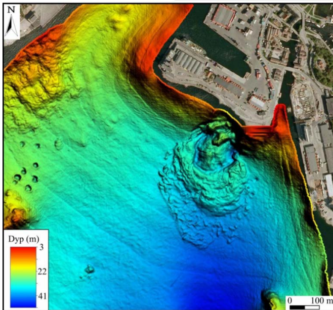
Figur 57: Undersjøisk skred (NGU)
