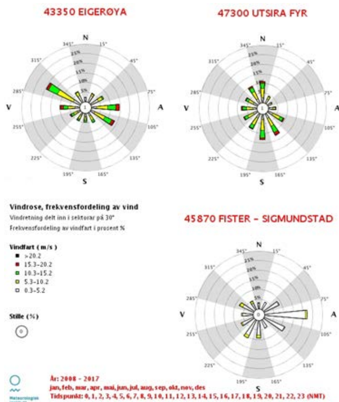
Figur 45: Vindroser frå perioden 2008-2017 (Kjelde: eKlima, 2018)
