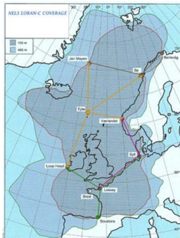
Figur 39: Loran C dekning og stasjonar (Kjelde: Nrk.no)
