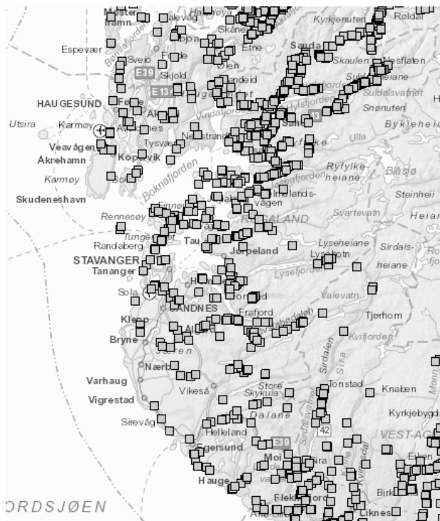
Figur 56: Registrerte steinskred/steinsprang i Rogaland i perioden 05.12.2010 -04.12.2017 (skredregistrering.no)
