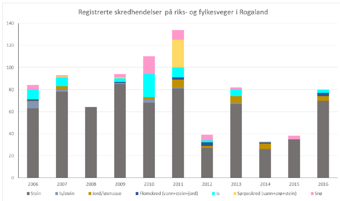
Figur 52: Registrerte skredhendingar på riks- og fylkesvegar i Rogaland 2006-2016 (Statens vegvesen, 2016a)
