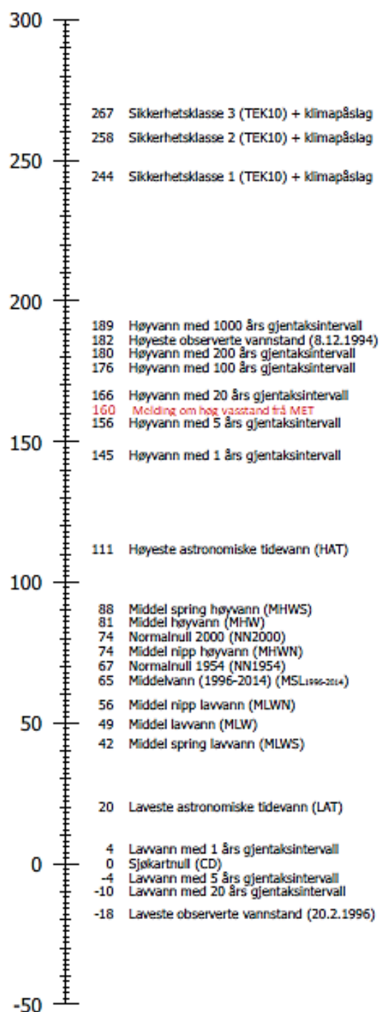
Figur 42: Nivåskisse med dei viktigaste vasstandsniåa og ekstremverdiar i Stavanger. Høgder er i cm over sjøkartnull (Statens kartverk, 2018b)
